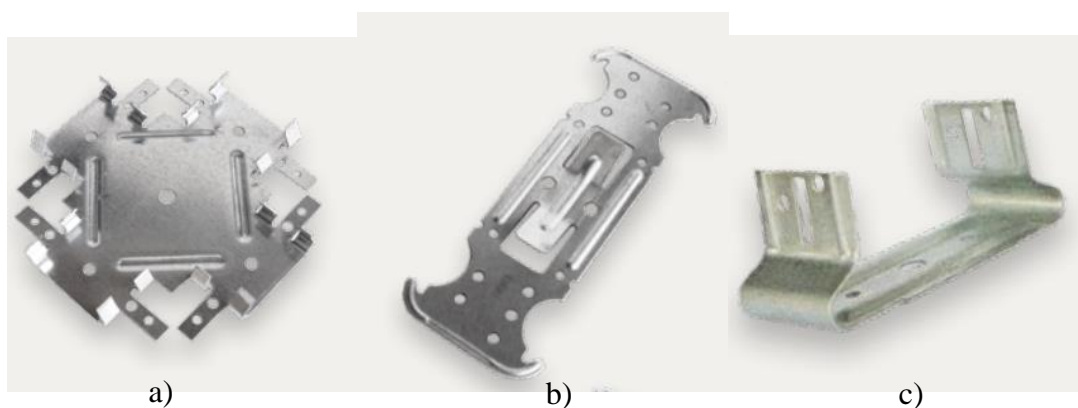
Slika 7. Montažni profili: a) nivo spojnica za CD profile b) križna spojnica – ravna za CD profile c) akustični ovjes [9]
