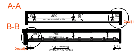
PRESJEK MJ 1:50
