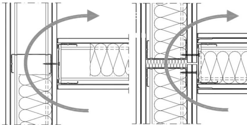
Slika 35. Spoj sa pregradnim zidom a) niska razina zvučne izolacije b) visoka razina zvučne izolacije (obradila Helena Frančić prema tehničkim detaljima iz „Knauf“ kataloga) [12]
