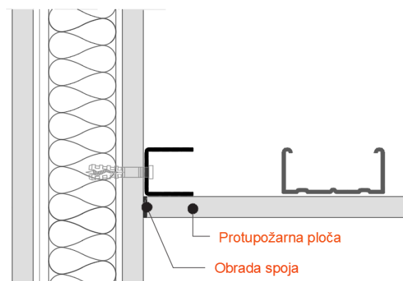
Slika 76. Protupožarni spojevi na pregradni zid (obradila Helena Frančič prema tehničkim detaljima iz „Knauf“ kataloga) [12]
