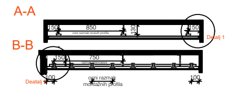
PRESJEK MJ 1:50
