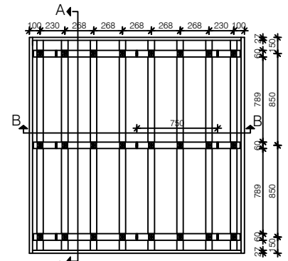
TLOCRT MJ 1:50
