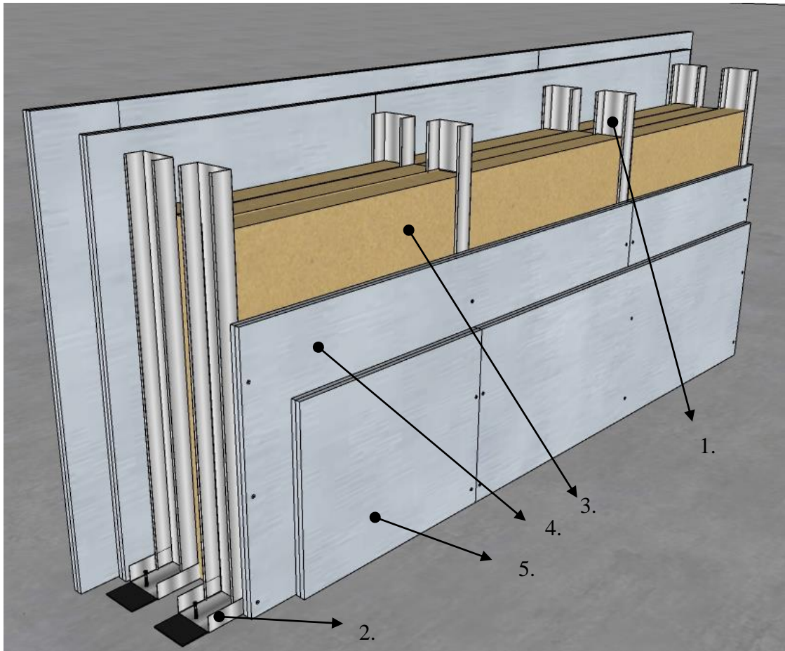
Slika 37. Pregradni zid visoke zvučne zaščite sa pločama Duo'Tech Rigips – 3D prikaz (crtala: Helena Frančič) [12]
