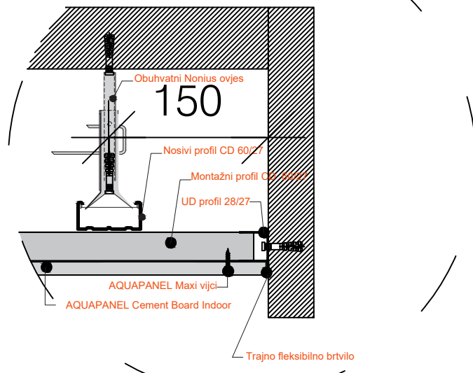
DETALJ 2 MJ 1:5
