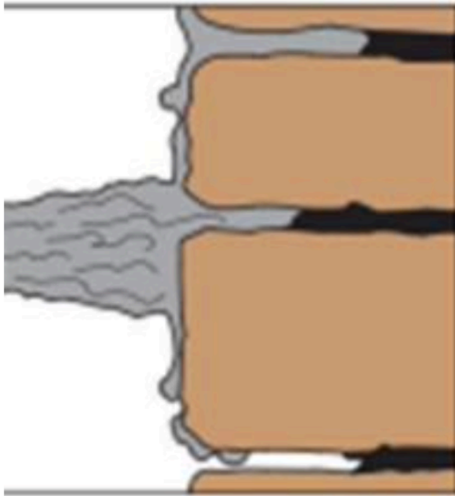
Slika 7.3. Zapunjavanje sljubnica
