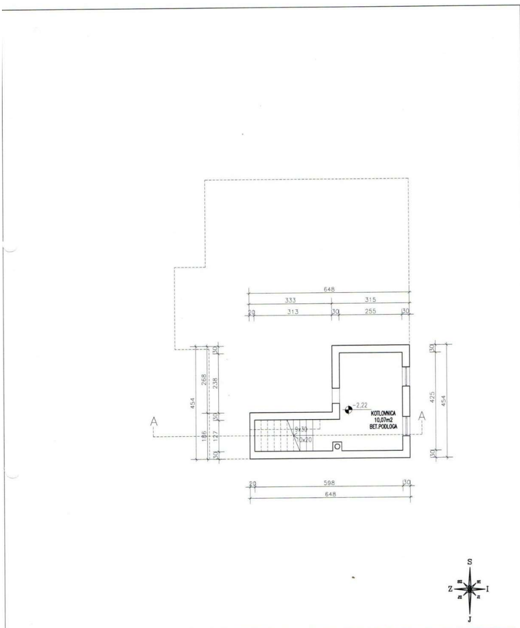
Slika 7. Tlocrt podruma
