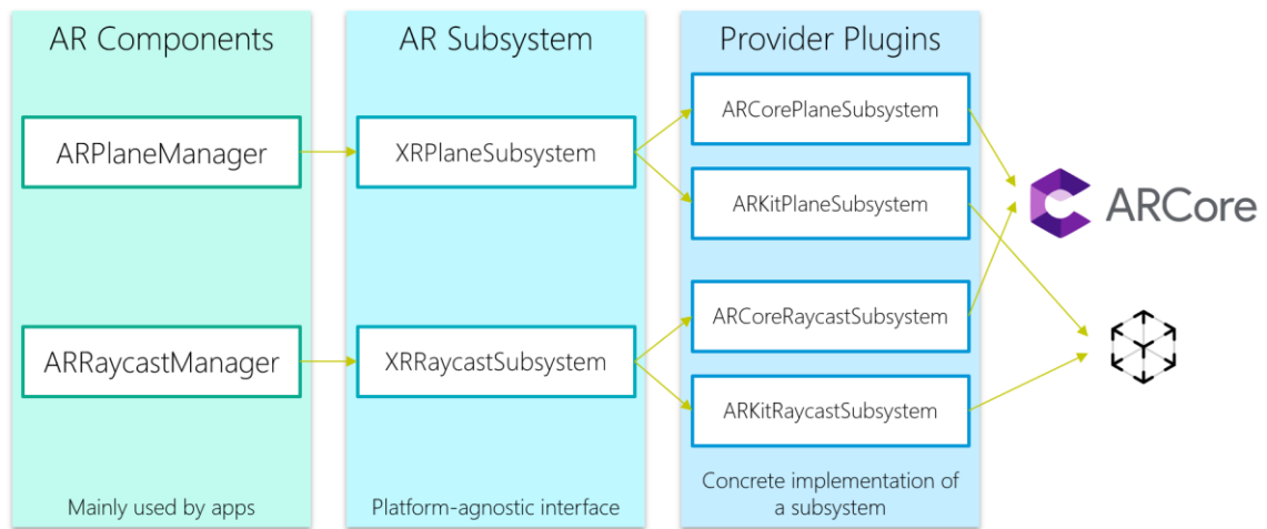
Slika 19: AR komponente, AR podsustav i okvir za dodatke u AR Foundationu
