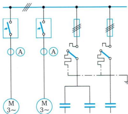
Slika 14. Grupna kompenzacija [5]
