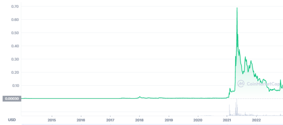
Slika 3 Grafikon DOGE-a 2015.-2023.
