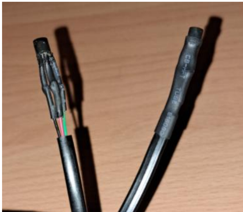
Slika 3.22. Prikaz senzora bez dodatnog bužira (lijevo) i vodootporni senzor sa duplim bužinom (desno)
