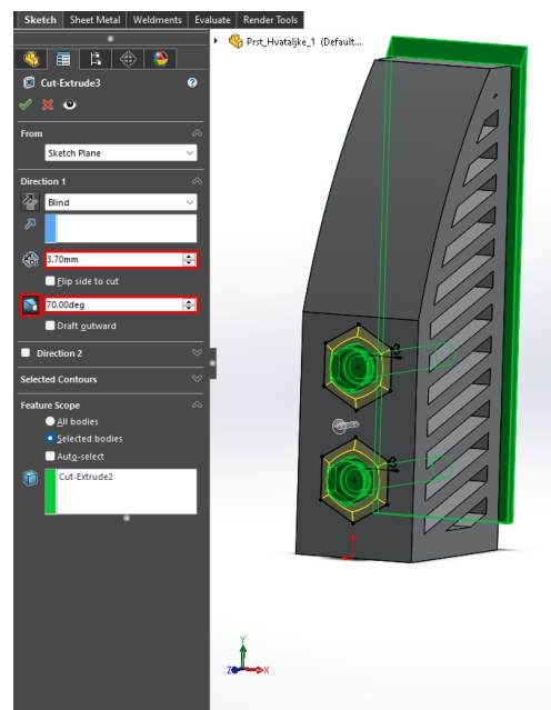
Slika 5.18. Proces zakosjenja glave vijka
