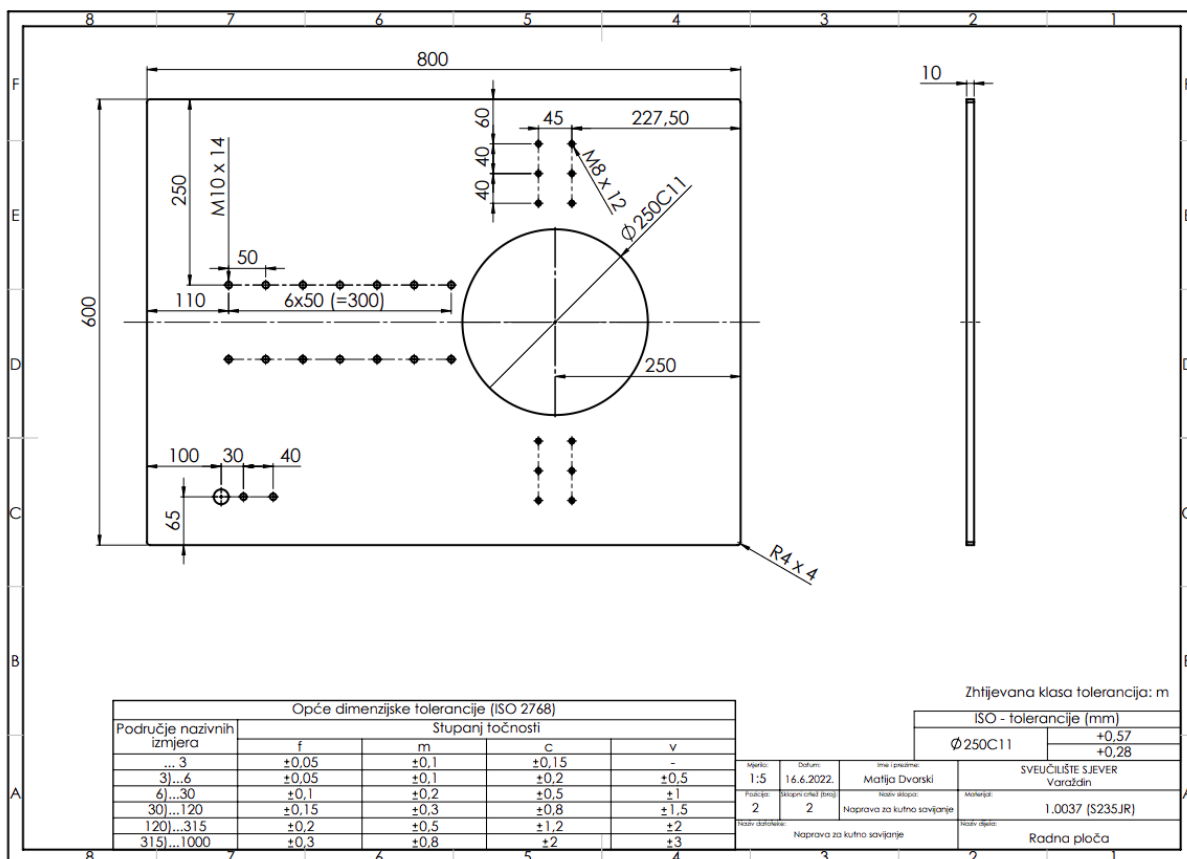
Slika 7.30: Tehnički crtež radne ploče
