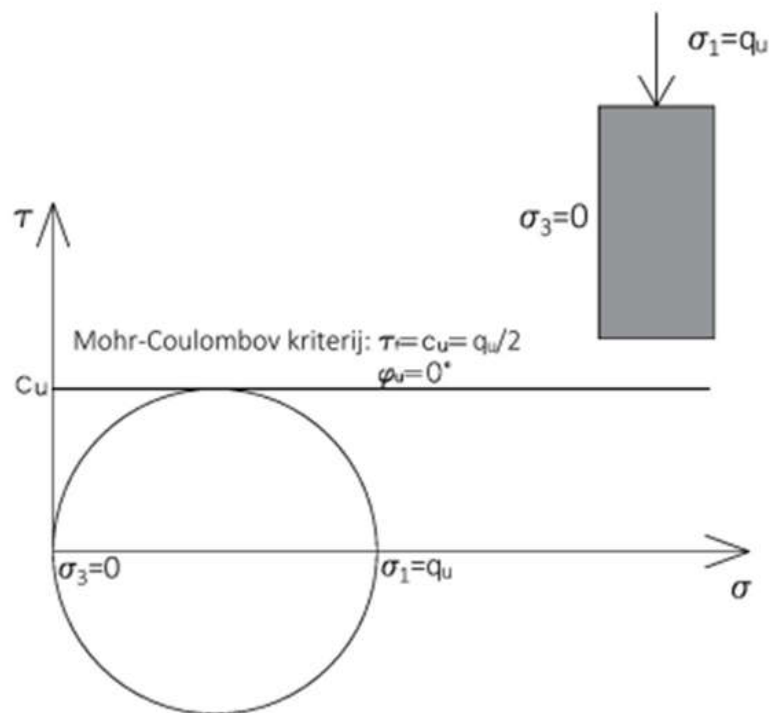
Slika 44.: Prikaz Mohrove kružnice za uzorak ispitan pokusom jednoosne tlačne čvrstoće, preuzeto iz [12]
