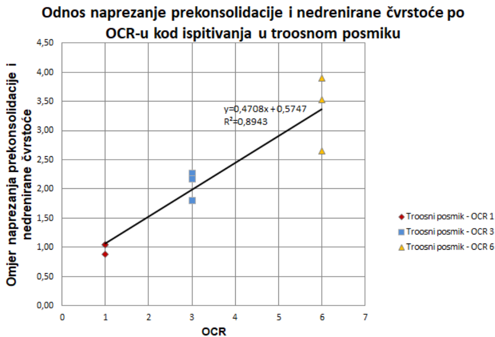
Slika 71.: Dijagram odnosa naprezanja prekonsolidacije i nedrenirane čvrstoće po OCR-u
