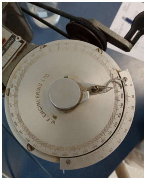
Slika 28.: Laboratorijska krilna sonda-mjerač kuta, (fotografirano uz dozvolu IGH, 2023.)
