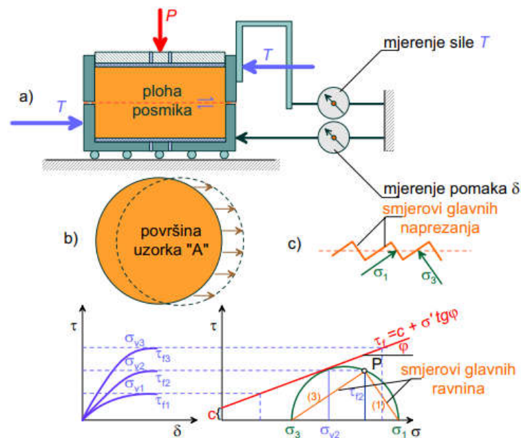
Slika 3. Presjek uređaja za izravni posmik i prikaz rezultata ispitivanja [4]
