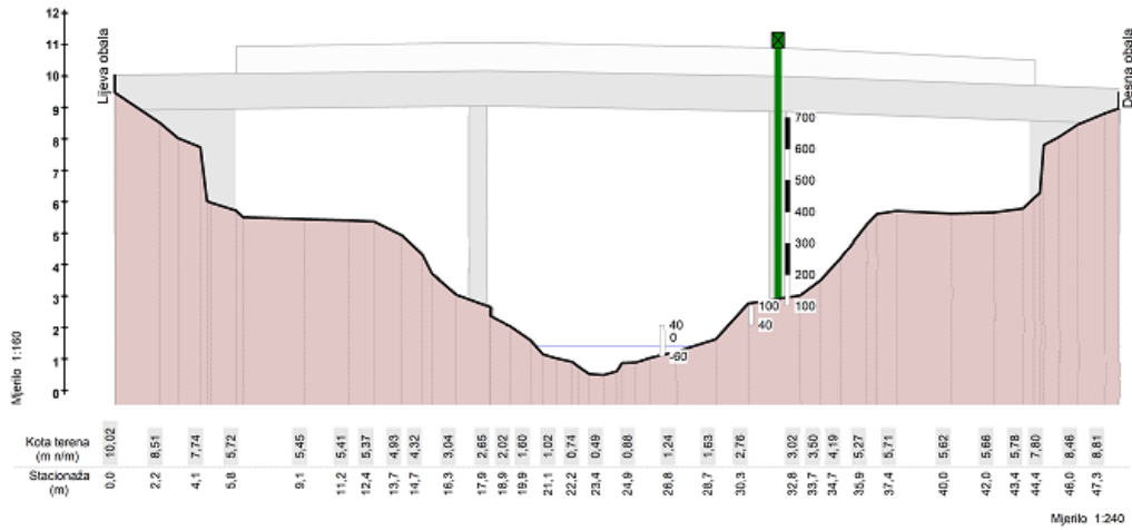
Slika 20: Poprečni presjek profila kod Motovuna [22]
