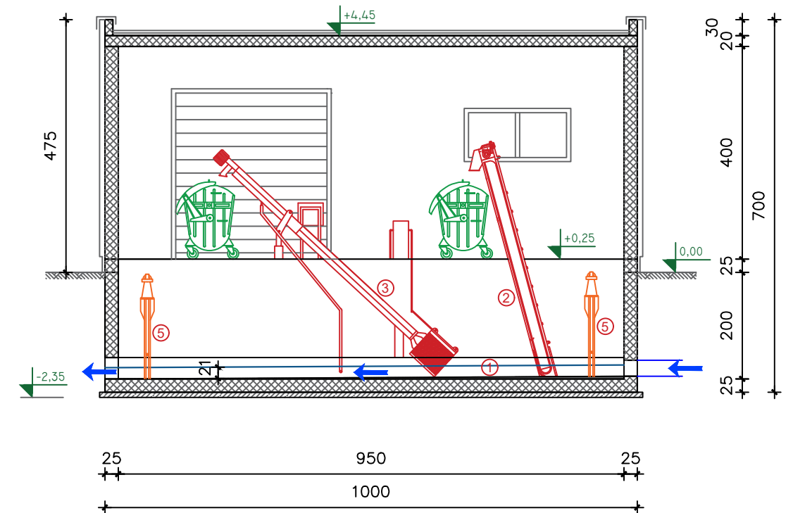
PRESJEK a-a
