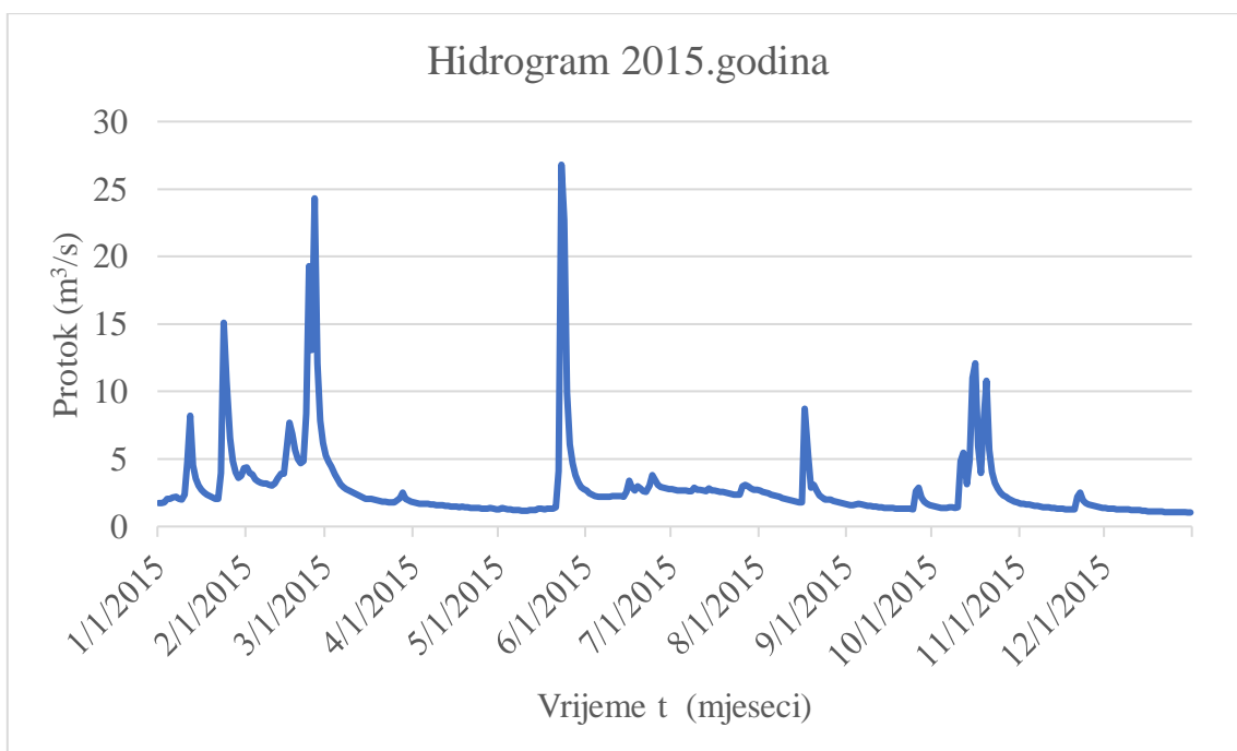
Slika 56. Hidrogram rijeke Plitvice u 2015. godini [5]
