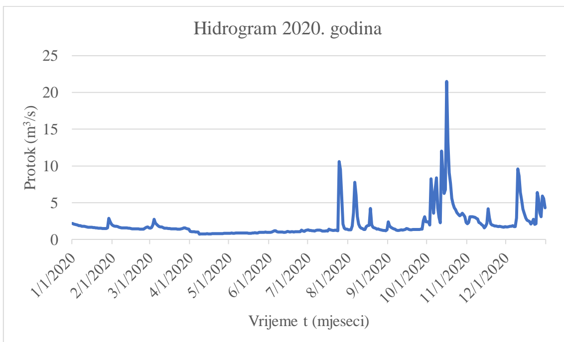
Slika 61. Hidrogram rijeke Plitvice u 2020. godini [5]
