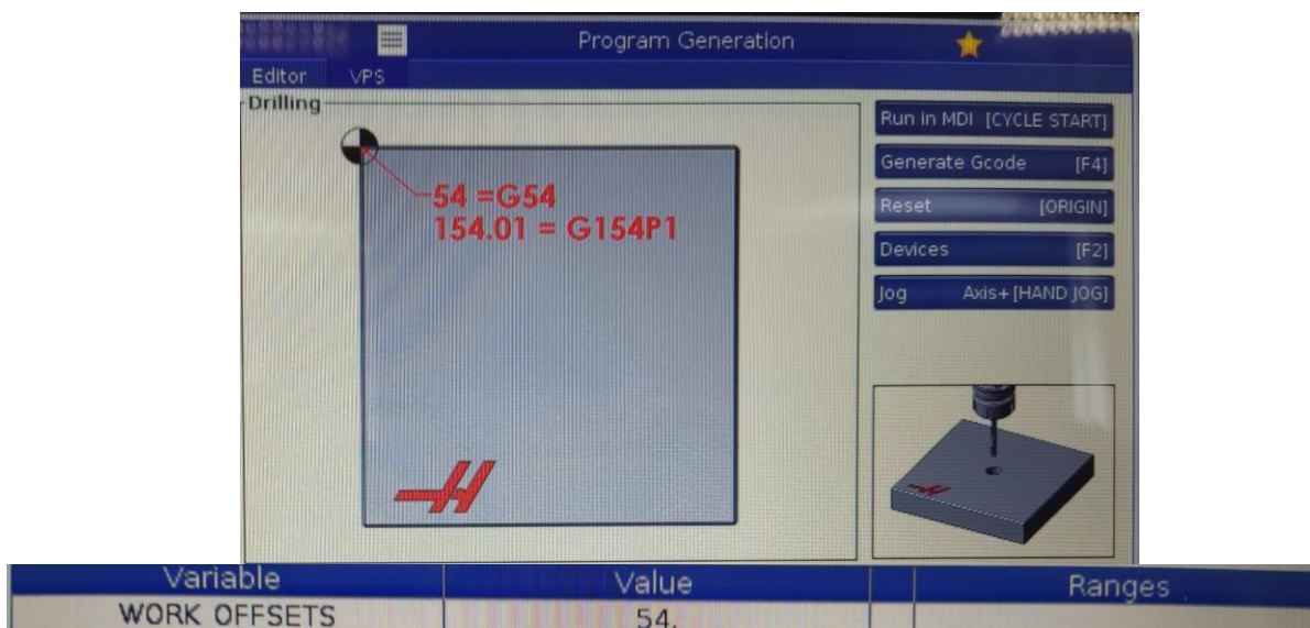
Slika 44. Nultočka obratka
