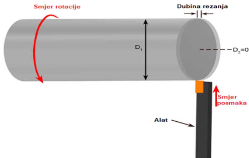
Slika 3 - Čeono tokarenje [4]
