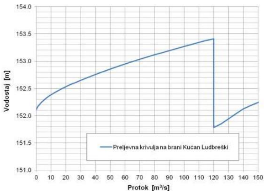
Slika 4.4. Preljevna krivulja brane Kućan Ludbreški u situaciji dizanja zapornica pri 120 m^3/s [8]
