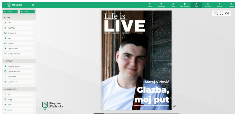
Slika 3.55. uređivanje flipbooka
