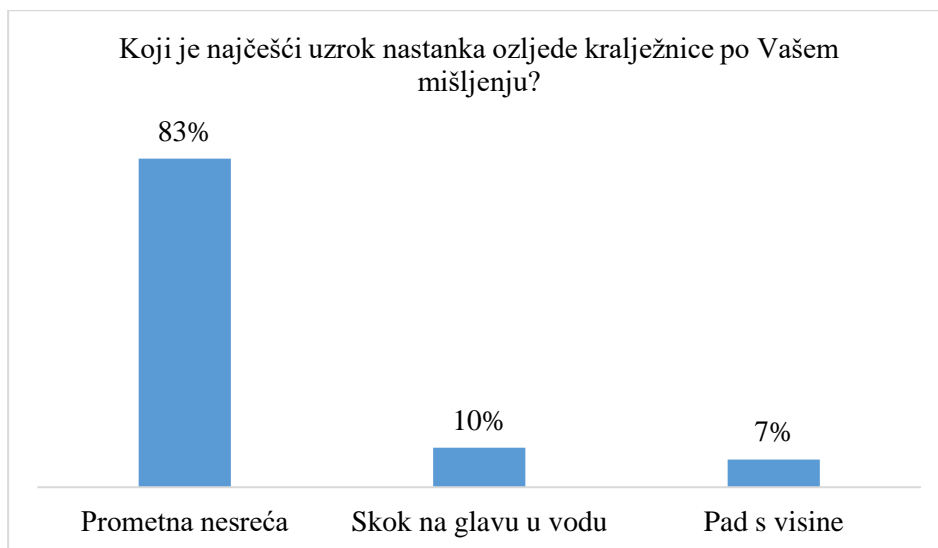
Grafikon 66.2 Najčešći uzrok nastanka ozljede kralježnice po mišljenju ispitanih
