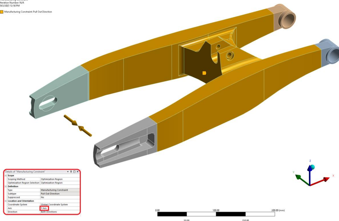
Slika 5.12 Smjer uklanjanja viška materijala
