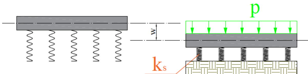
Slika 4.2. Jednoparametarski model tla
