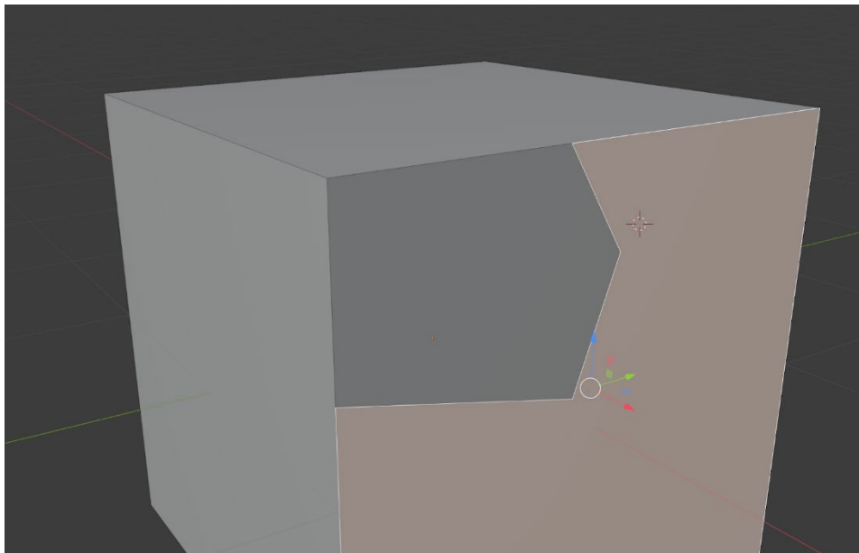
Slika 2.3: N-gon
