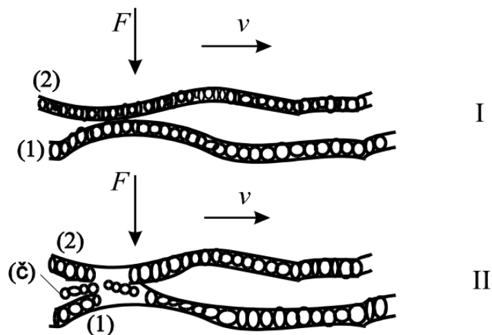
Slika 3.5. Faze tribokorozije [13]
