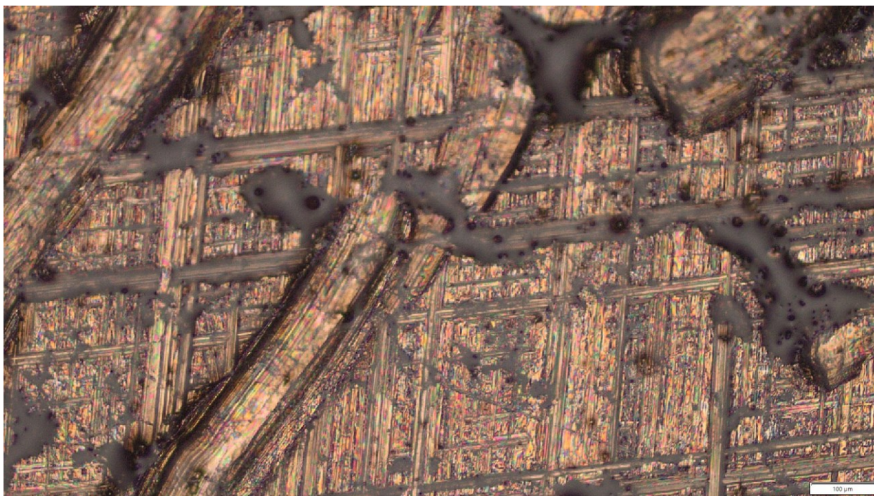
Slika 7.6. Uvećanje pločice S235JR x100 manje bruniranog mjesta na pločici
