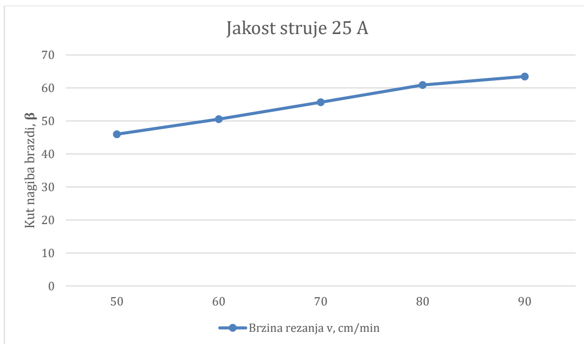
Slika 22. Ovisnost kuta nagiba brazdi o brzini rezanja kod jakost struje 25 A
