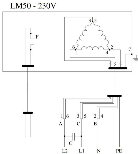
Slika 3.1.2. Shema spajanja linearnog motora [4]
