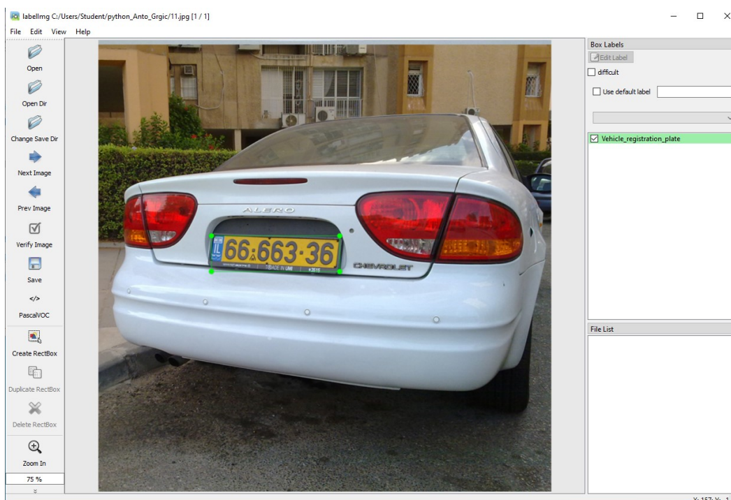
Slika 8.1. LabelImg
