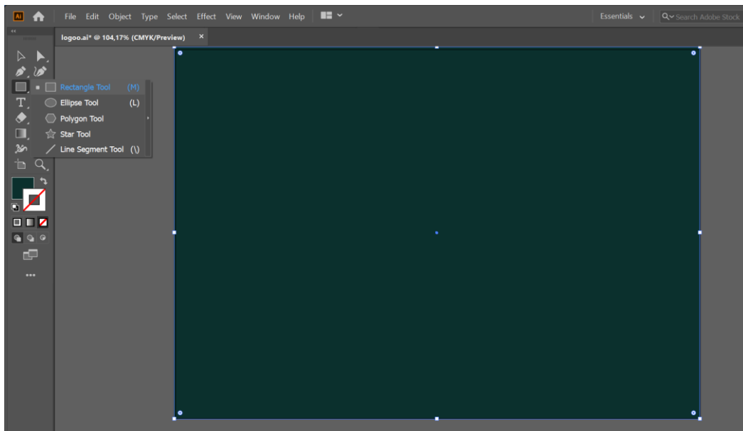
Slika 18 Izrada pozadine
