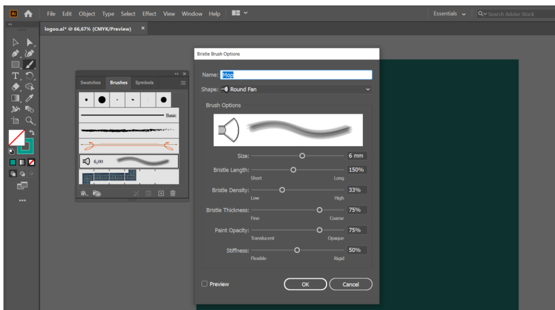
Slika 19 Izrada kista
