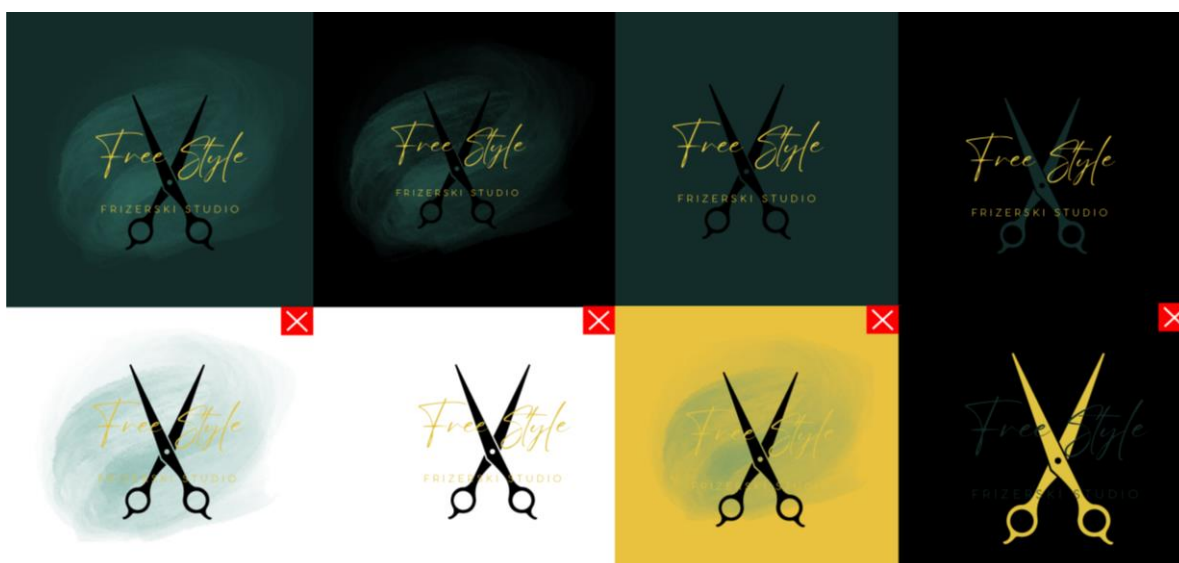
Slika 29 Varijante loga
