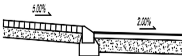
Slika 74. Rubnjak između kružne trake i voznog dijela središnjeg prometnog otoka [17]
