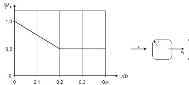
Slika 10.19. Faktor smanjenja za kvadratne profile sa zaobljenim rubovima (drvo nema zaobljene rubove, radijus =0) Faktor smanjenja \Psi_r = 1,0
