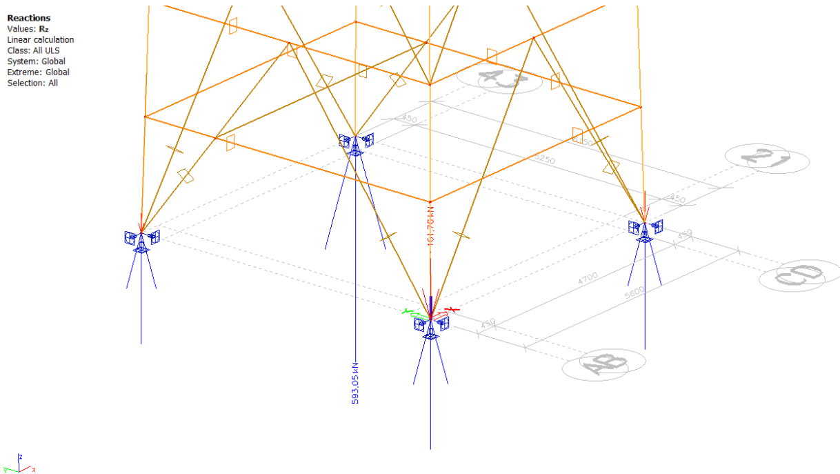
Slika 10.21. Model konstrukcije s reakcijom ležaja na vrhu temelja
