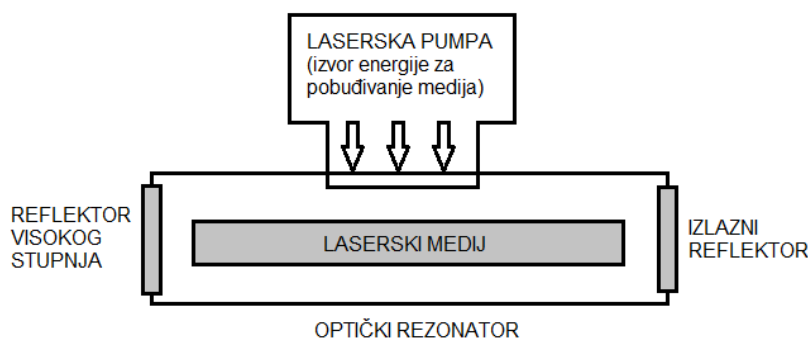
Slika 7. Građa lasera [1]
