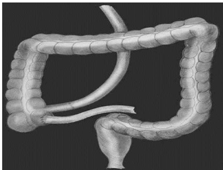
Slika 1.1.1. Jejunum-ilealna prenosnica
