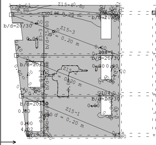
Okvir V_8 Aa - d.zona - Pravac 1 - max Aa1,d= 4.02 cm 2 /m
