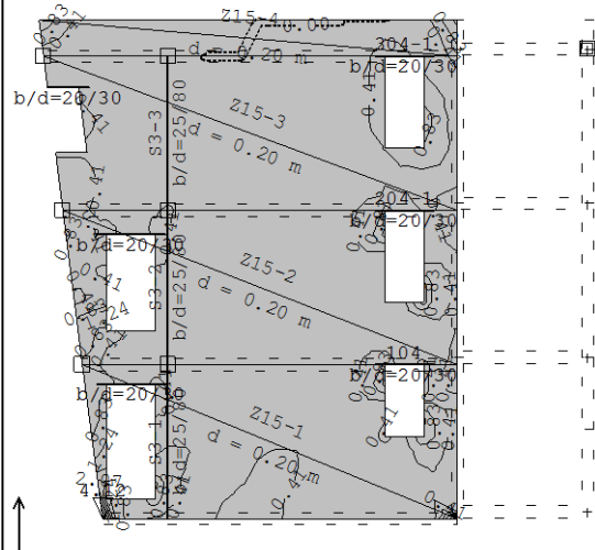
Okvir V_8 Aa - d.zona - Pravac 2 - max Aa2,d= 4.12 cm 2 /m
