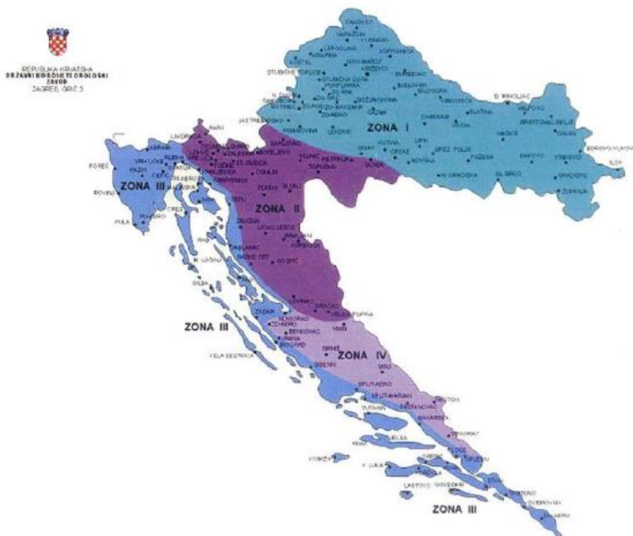
Slika 2.3.1 Klimatske zone karakterističnog opterećenja snijegom[3]
