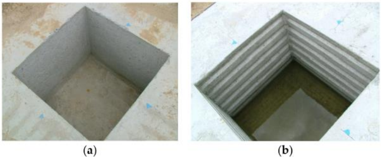
Slika 3.1 Prikaz unutarnje površine temeljnih čaša: (a) s glatkom površinom i (b) s nazubljenom površinom [4]
