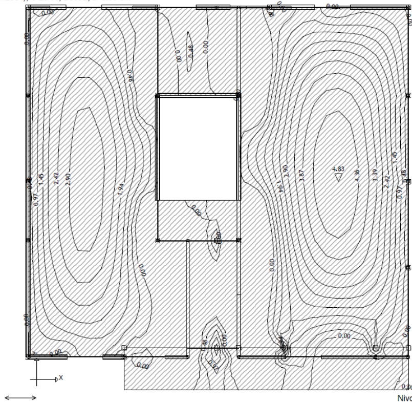
Nivo: strop prizemlja [3.16 m] Aa - d.zona - Pravac 1 - max Aa1,d= 4.83 cm 2 /m
