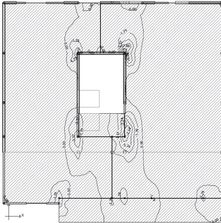
Nivo: strop kata [6.19 m] Aa - q.zona - Pravac 1 - max Aa1,g= -17.86 cm 2 /m
