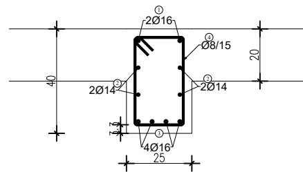
G206 PRESJEK 1-1 M: 1:50
