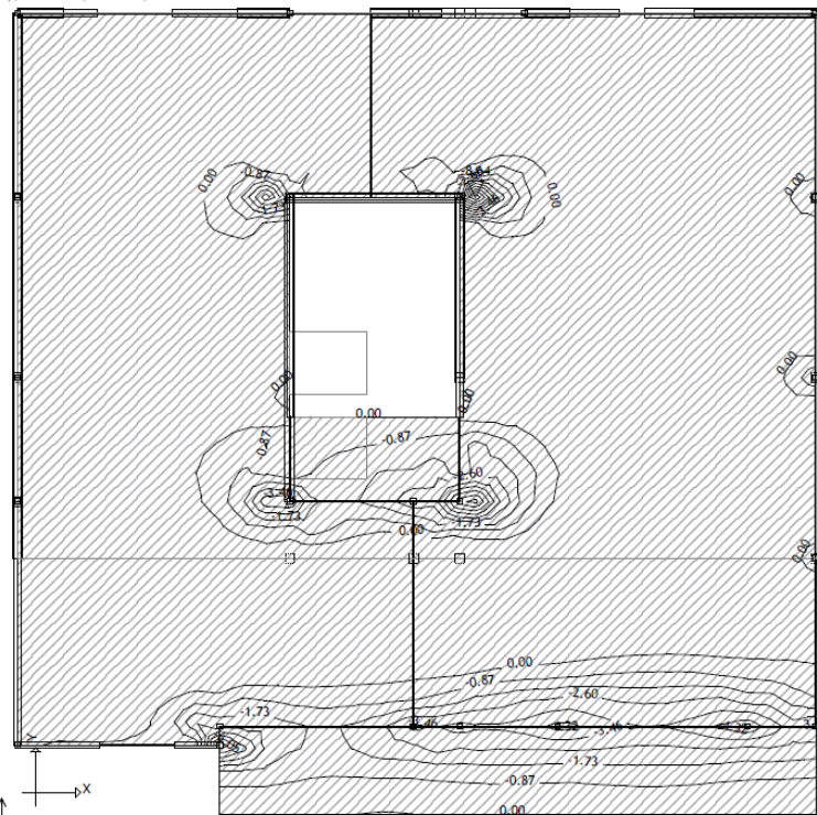
Nivo: strop kata [6.19 m] Aa - q.zona - Pravac 2 - max Aa2,g= -8.64 cm 2 /m
