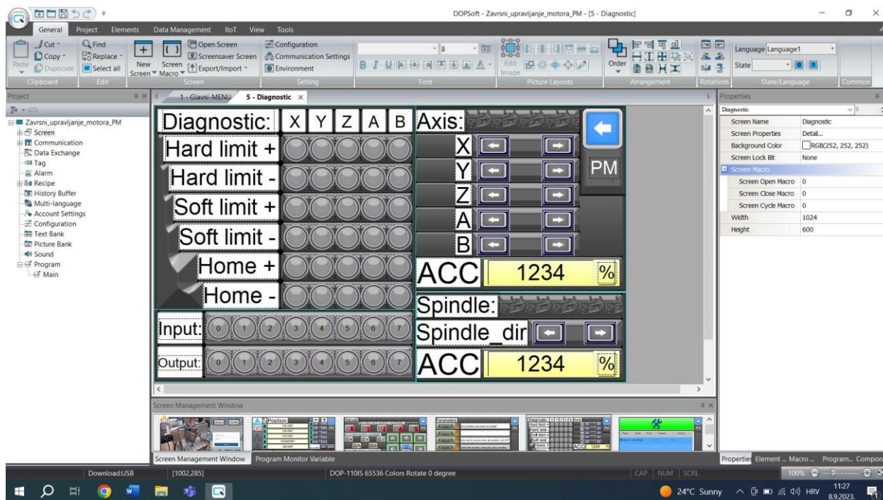
Slika 5.23 Numerički unos [6]
