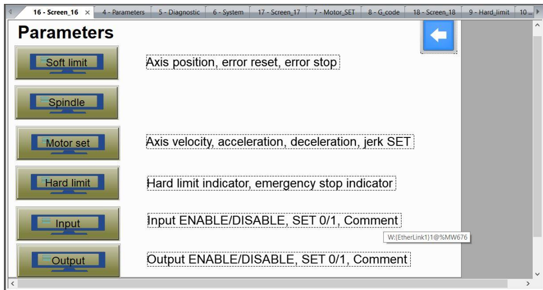
Slika 5.20 Parametri
