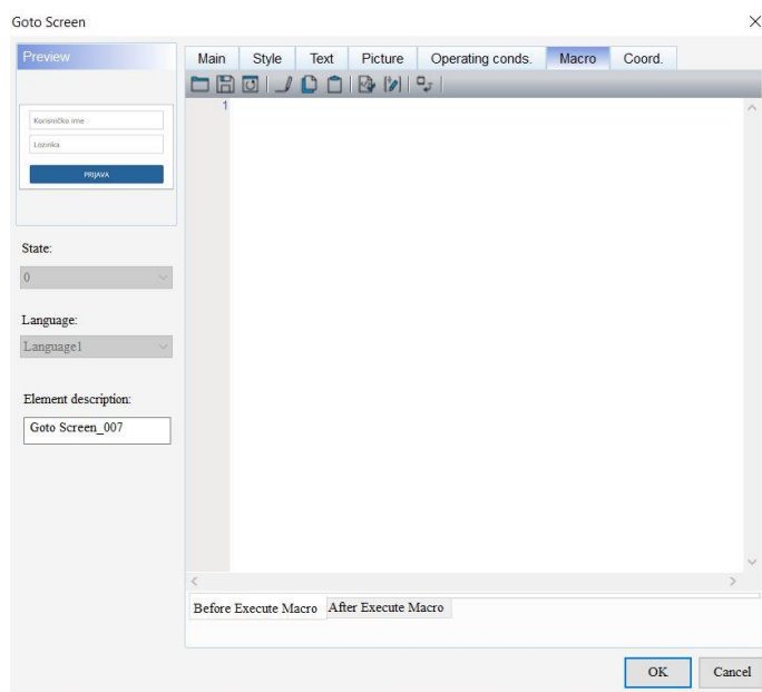
Slika 5.5 Postavljanje macro
