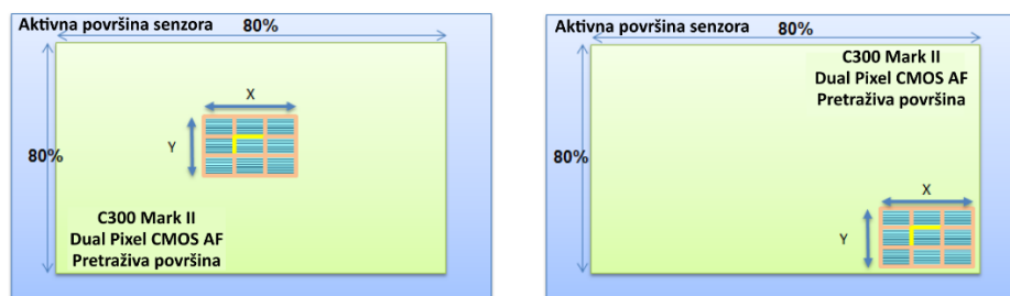
Slika 5.13 - Mogućnost pomicanja područja senzora koje će se koristiti za automatsko fokusiranje kod kamere C300 Mark II [52]
