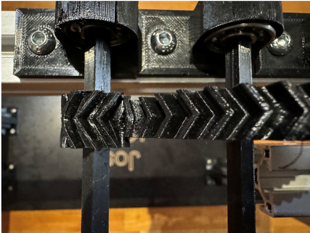
Slika 29 Prikaz dvaju zupčanika u zahvatu
