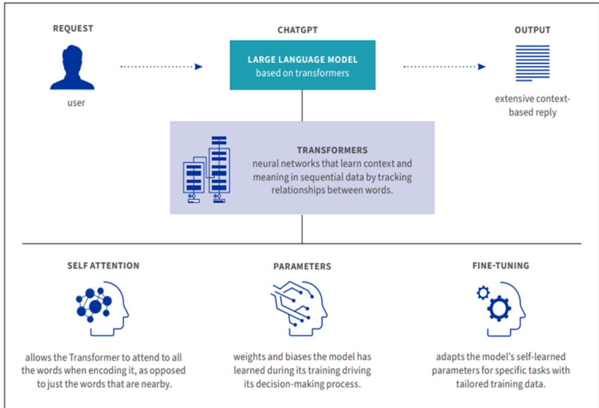
Slika 4. Funkcioniranje ChatGPT-a
