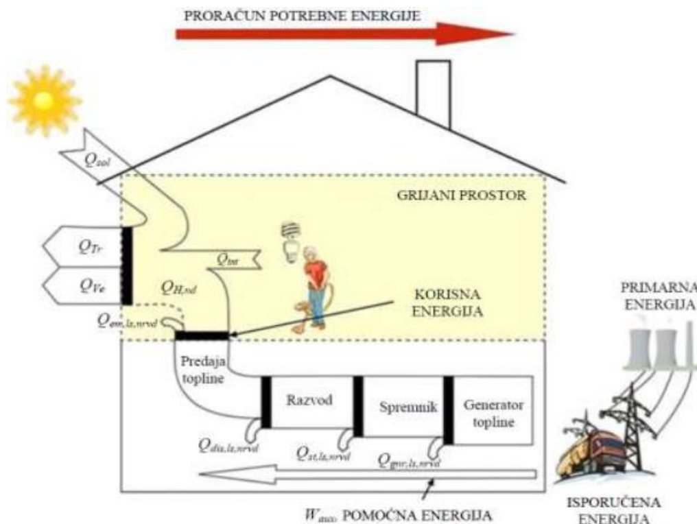
Slika 2.4.1; Tokovi energije [10]
