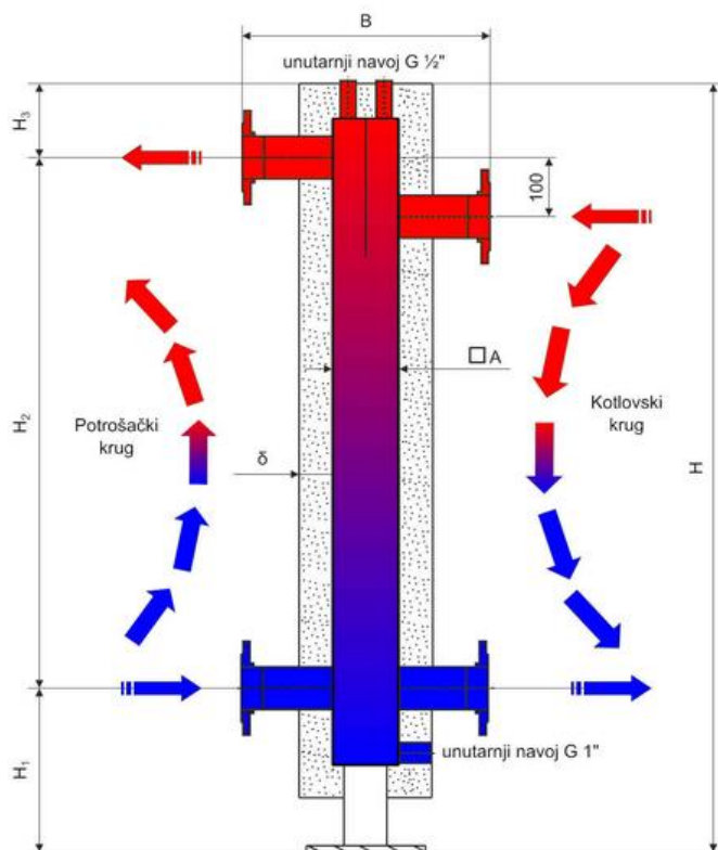
Slika 5.3.1; Hidraulička skretnica [14]
