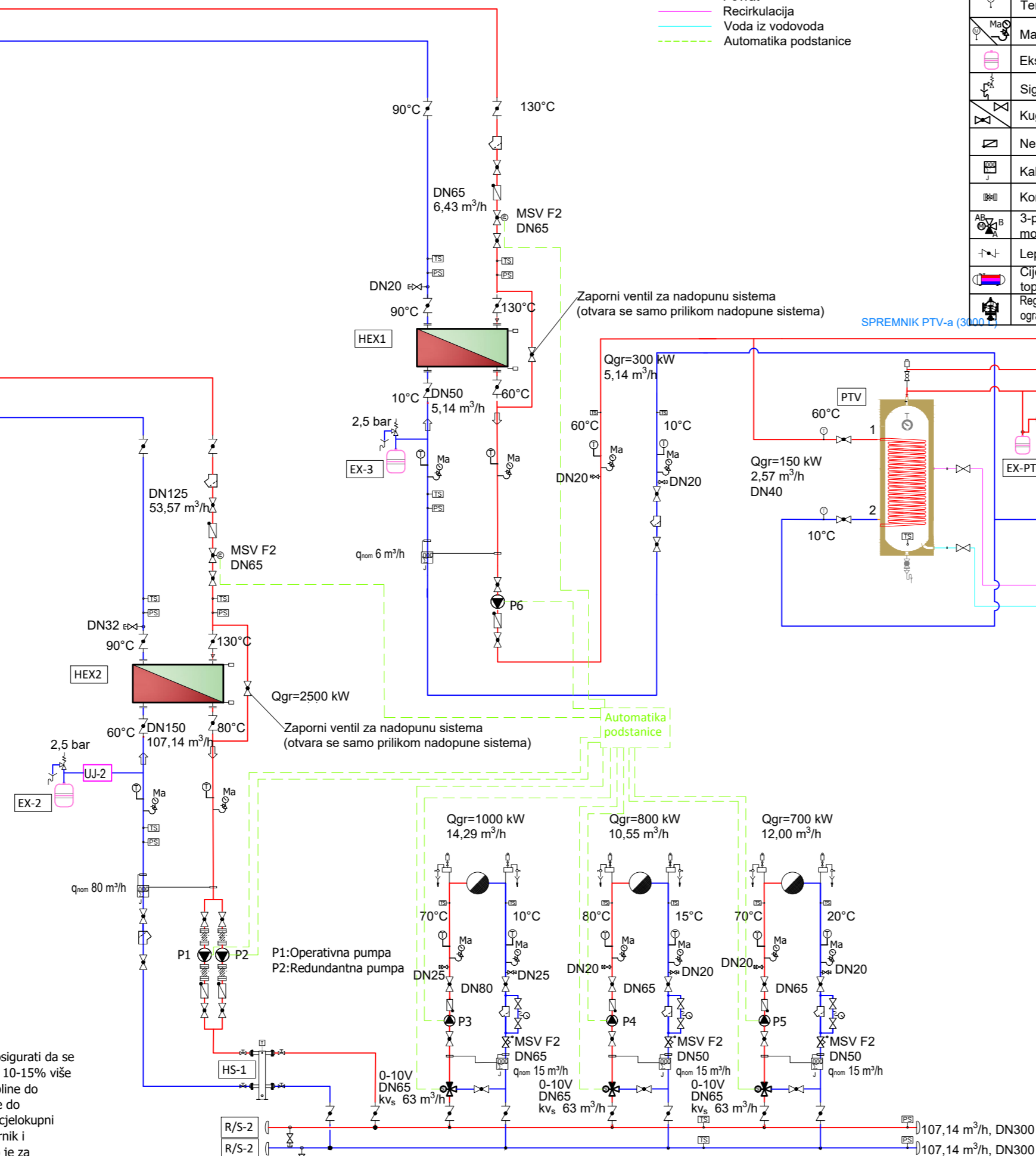
Prilog br. 21 Hidraulička shema indirektnog sustava grijanja i PTV-a (pločasti izmjenjivač) [autor]
