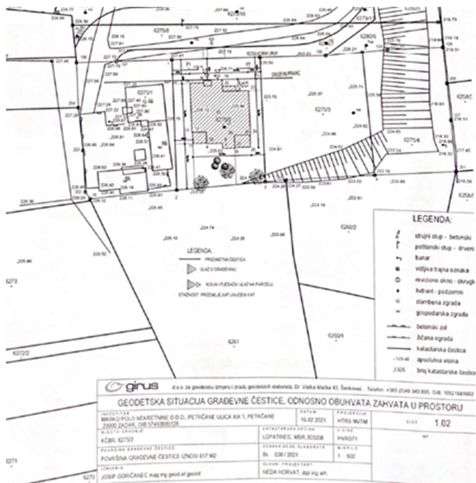
Slika 2.1.1. Geodetska situacija građevne čestice
