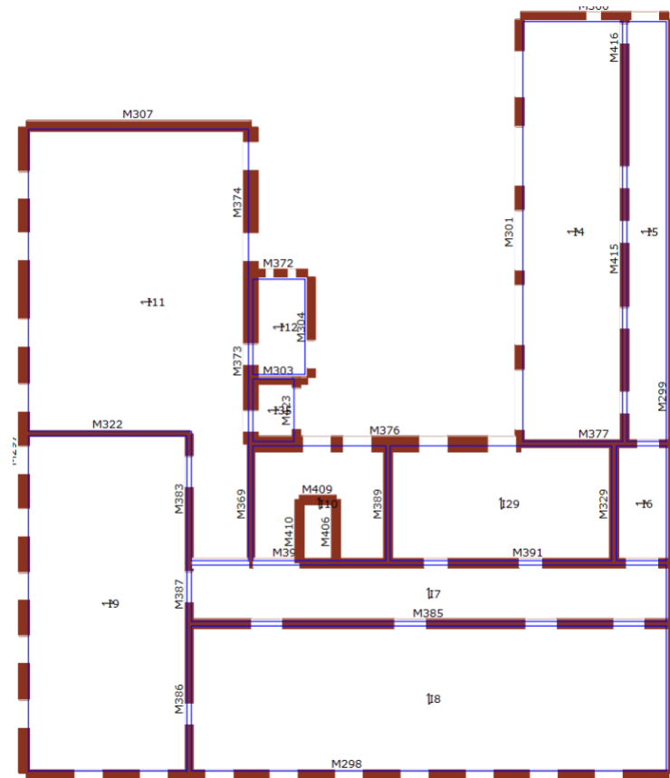
Slika 8.4 Tloerť 1. kata (grafiki prikaz razine iz programa 3Muri)
