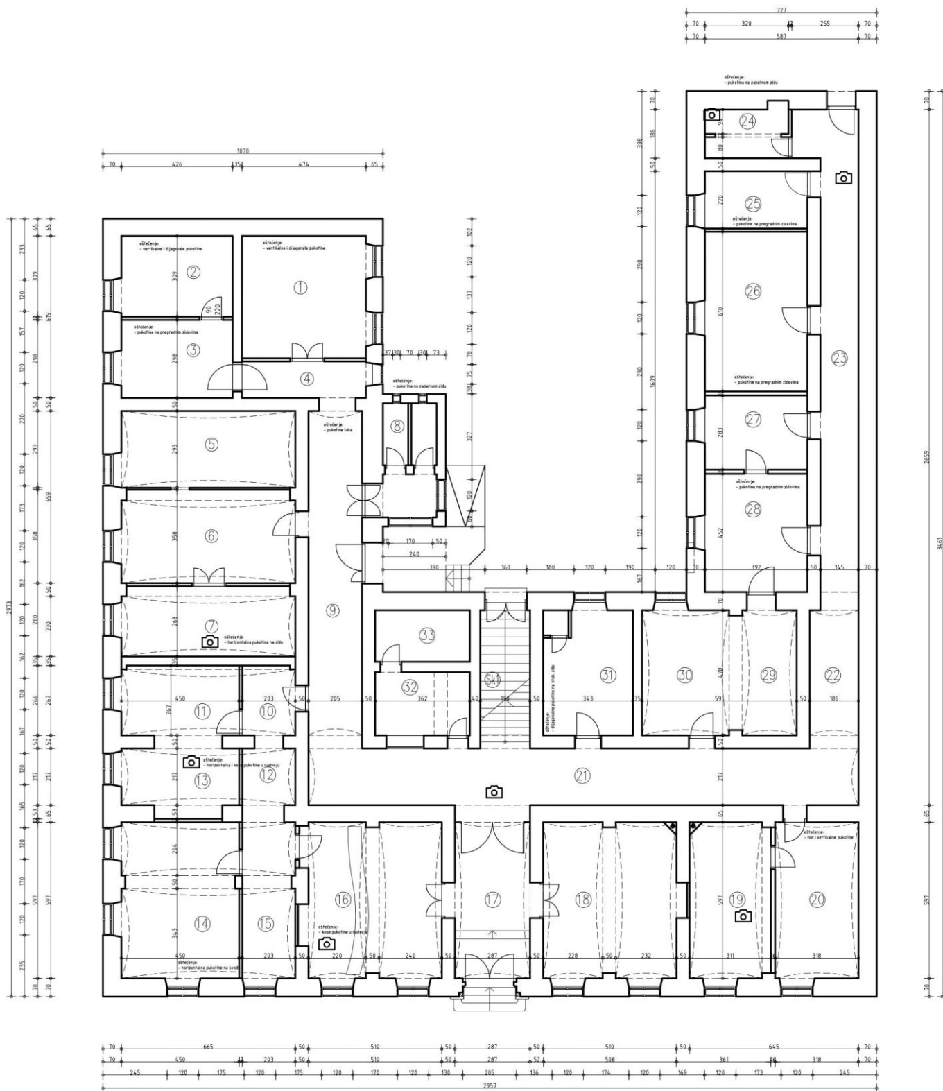
POSTOJEĆE STANJE TLOCRT PRIZEMLJA 1:200
