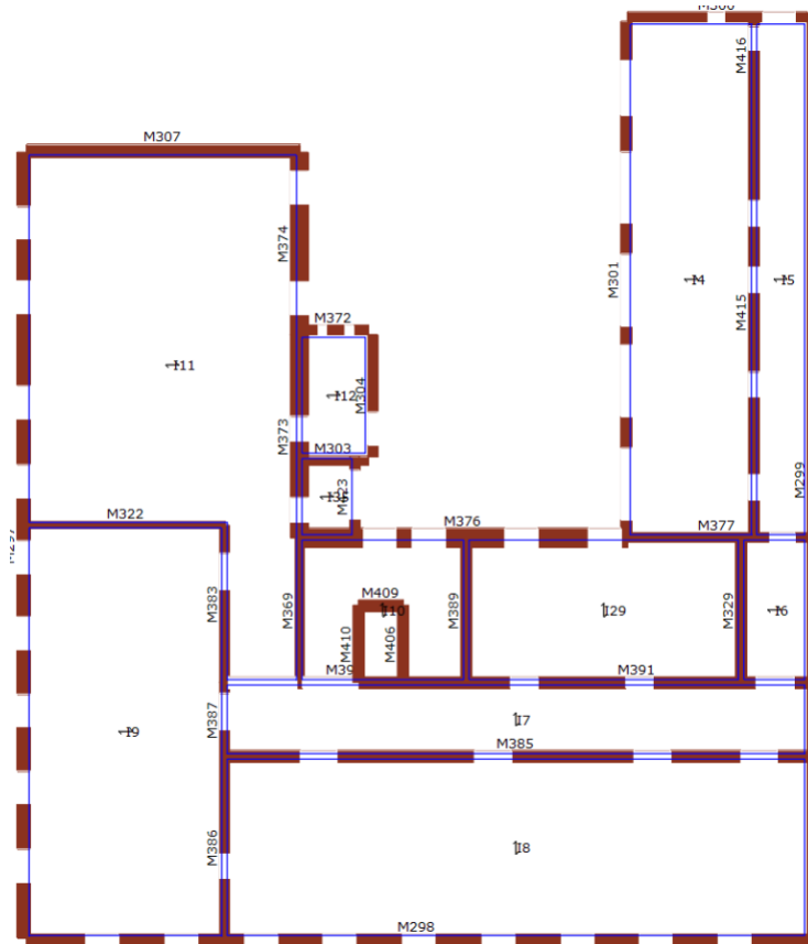
Slika 8.4 Tloerc 1. kata (grafički prikaz razine iz programa 3Muri)
