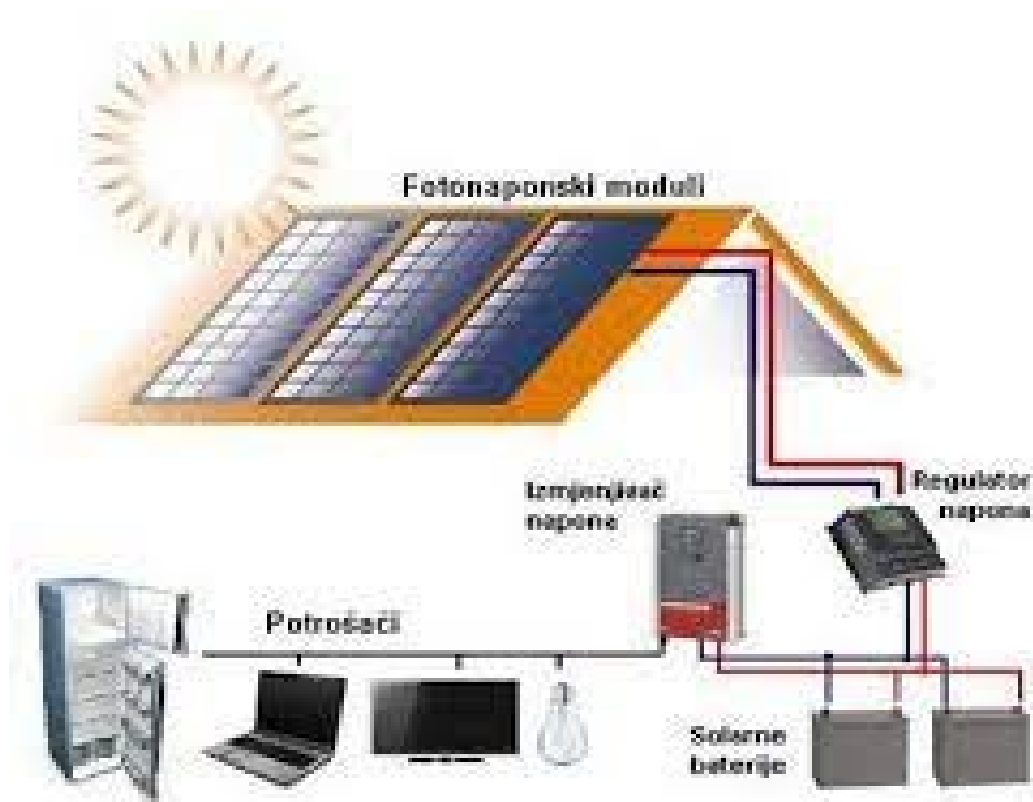
Slika 13. Samostalni fotonaponski sustav [10]
