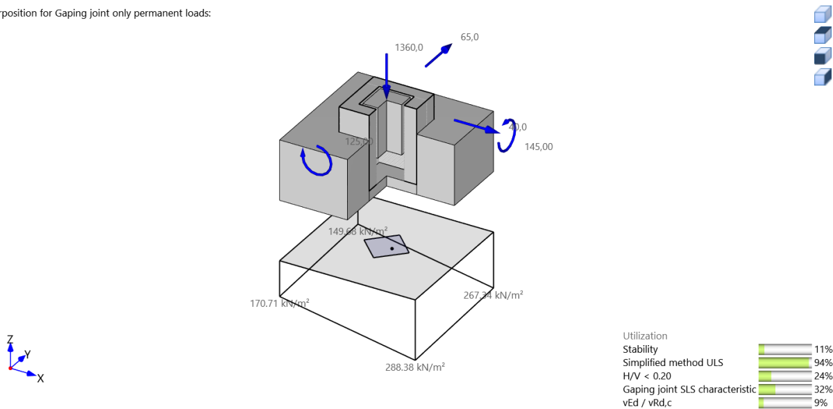
Slika 3.111. Prikaz kontaktnih naprezanja
