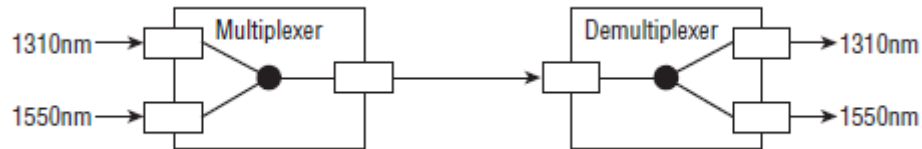
Slika 2.5. Širokopolasni WDM sustav [1]
