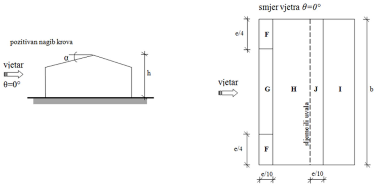
Slika 3.3.2.2. Podjela dvostrešnog krova po zonama za transversalni smjer vjetra
